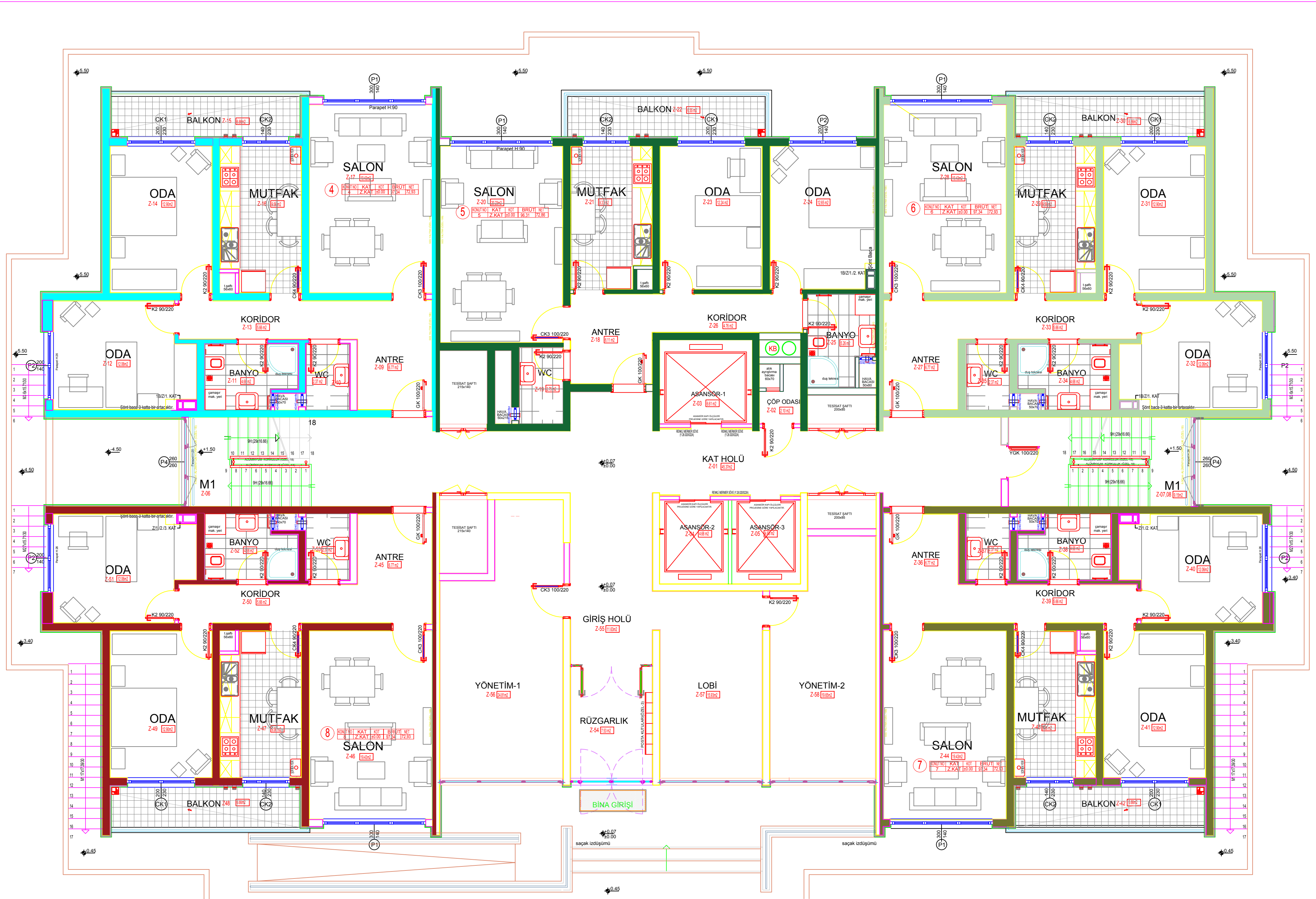
ANKARA SİNCAN SARAYCIK MAHALLESİ G.Ö.B. KENTSEL DÖNÜŞÜM PROJESİ SF TİP BLOK ZEMİN KAT PLANI
